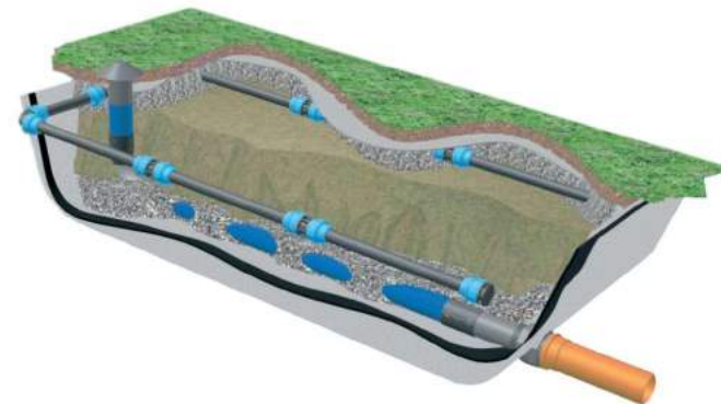
OPBYGNING AF BIOLOGISK SANDFILTERANLÆG
