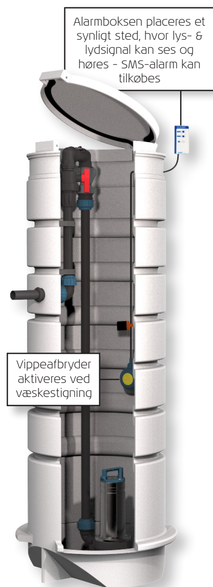
Eksempel på Ø600 spildevandsbrønd med VA-alarm
